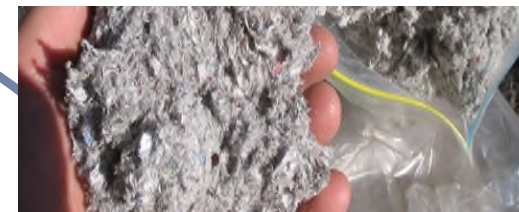
Cellulose
