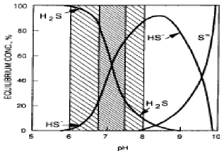
FIGUUR 2-1 DE PH AFHANKELIJKHEID VAN HET EVENWICHT TUSSEN \text{H}_2\text{S} , \text{HS}^- EN \text{S}^{2-} , GEBASEERD OP (RINTALA & PUHAKKA 1994).
