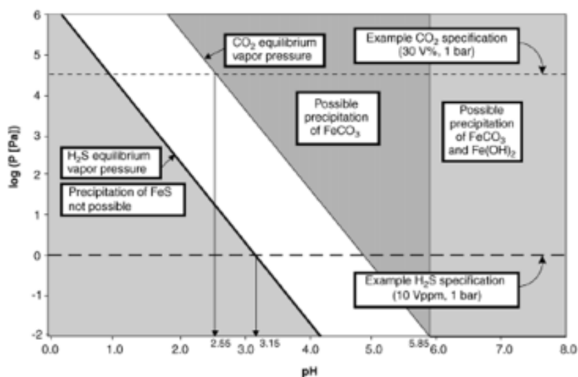
FIGUUR 2-2 DAMPSpanning van CO 2 en H 2 S als functie van de pH van een 1M FeSO 4 -oplossing bij een temperatuur van 293 K. De onderbroken lijnen is de H 2 S uitgaand specificatie (10 ppmv bij 1 bar) en the CO 2 dampspanning in het ingaande gas (30 vol.% bij 1 bar) (ter maat 2005).
