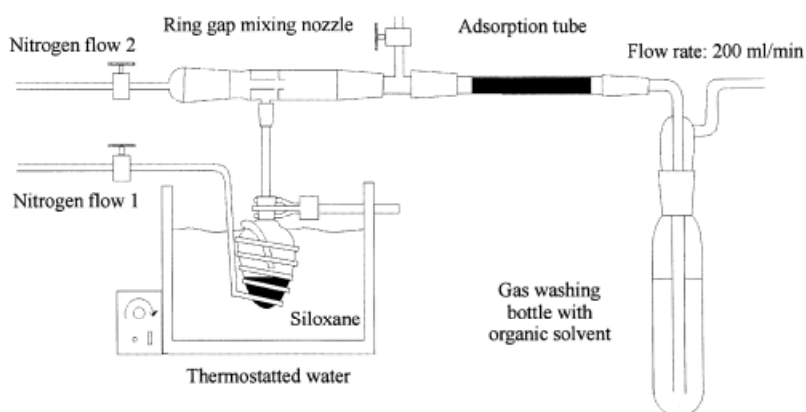
FIGUUR 4-2 PROEFOPZET VOOR HET GENEREREN VAN TESTGAS EN ADSORPTIE/ABSORPTIE EXPERIMENTEN.
