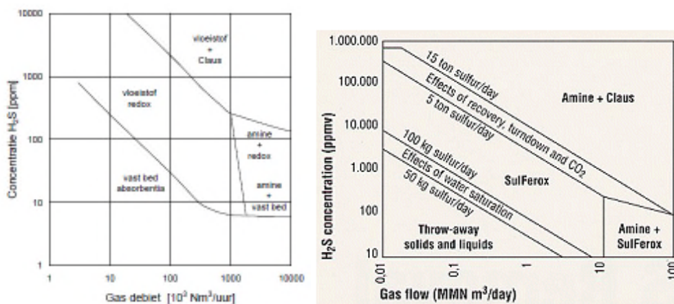
FIGUUR 2-6 TOEPASSINGSGBIED VAN TECHNIKEN VOOR S-VERWIJDERING (LINKS: CARNELL & WOODWARD, RECHTS: KLINCENBIJN ET AL. 1999).
