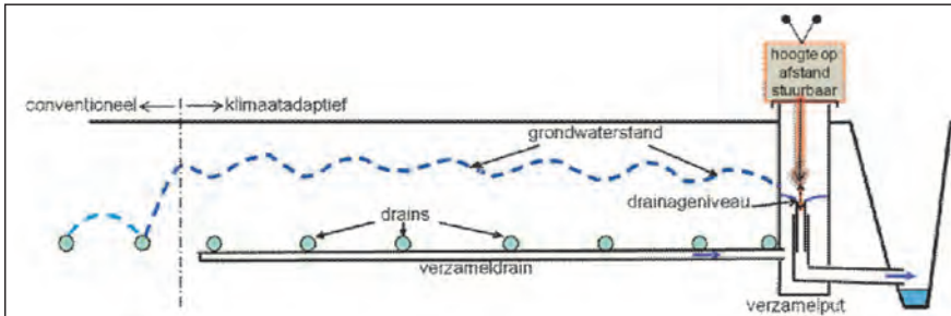
Afbeelding 1: Klimaat Adaptieve Drainage (KAD) systeem: drains, verbonden met een gesloten verzamelrain, die uitkomt in een verzamelput met automatisch gestuurd drainageniveau, en een afvoerleiding naar het oppervlaktewater.
