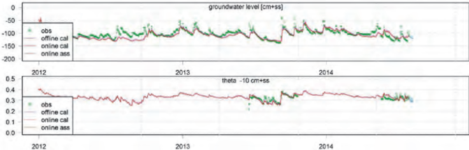
Afbeelding 8: Voorbeeld van gemeten en gesimuleerde (na kalibratie en assimilatie) grondwaterstanden (boven) en bodemvochtgehaltes (onder), voor het KAD-perceel in Haaksbergen.
